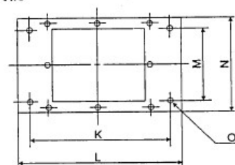
A-A矢視
