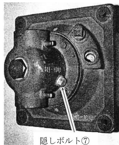
隠しボルト設置状況 (HT-100K、200K、400K)
