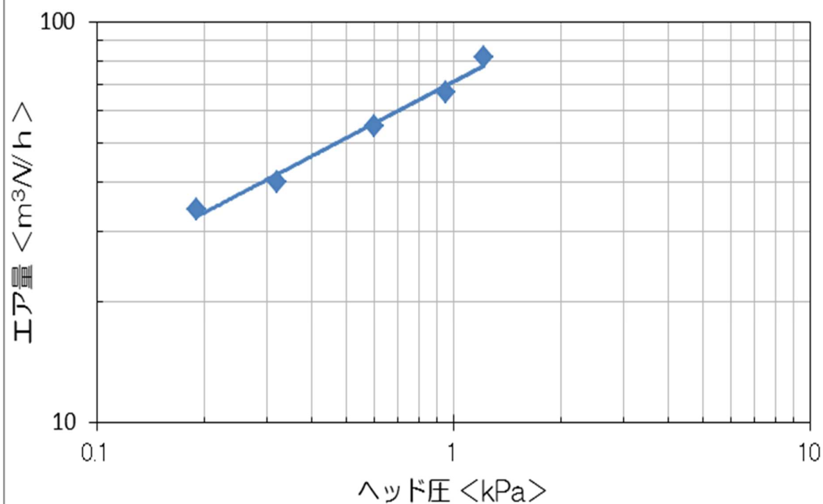
【エア量とヘッド圧】※ オープン燃焼
