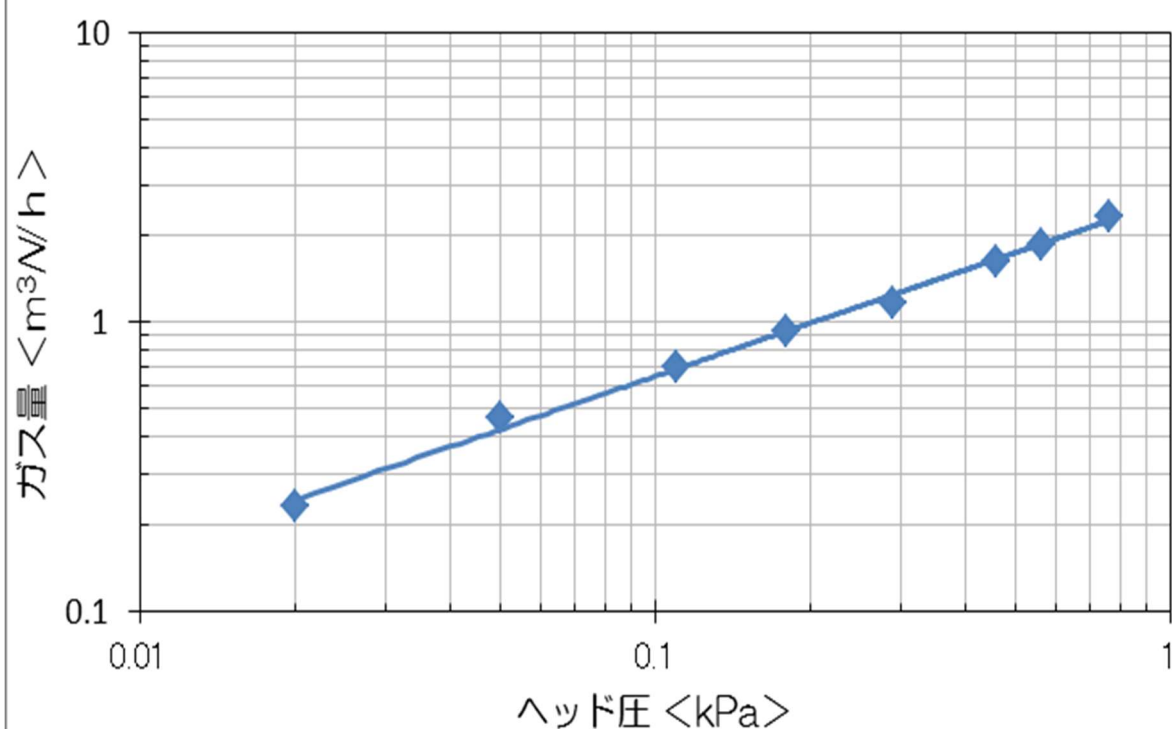
【ガス量とヘッド圧】※ オープン燃焼
