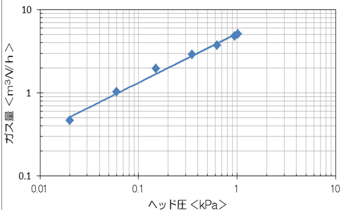
【ガス量とヘッド圧】※ オープン燃焼
