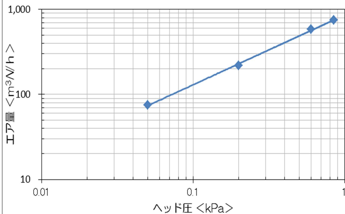
【エア量とヘッド圧】※ オープン燃焼
